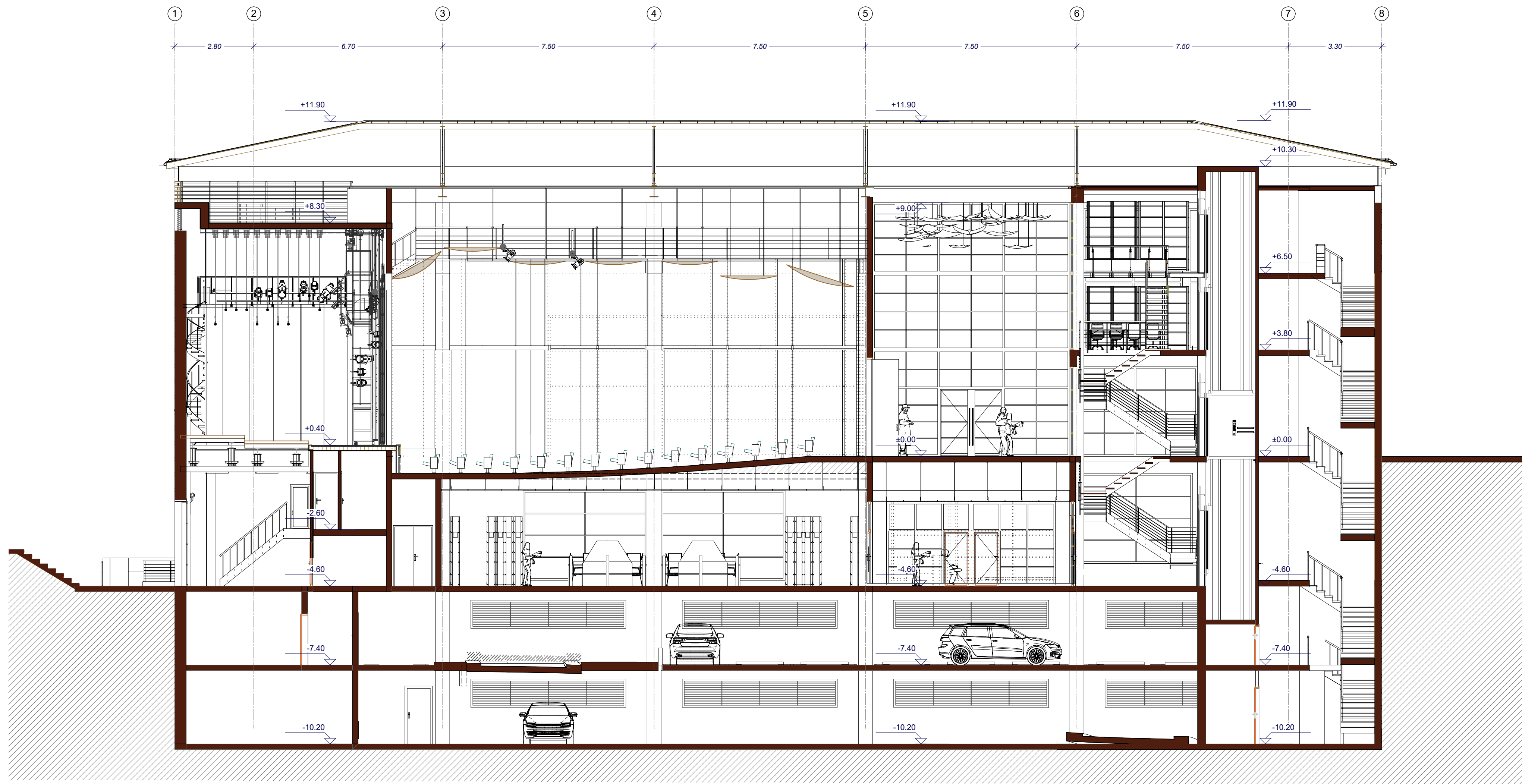
ΤΟΜΗ Α-Α
