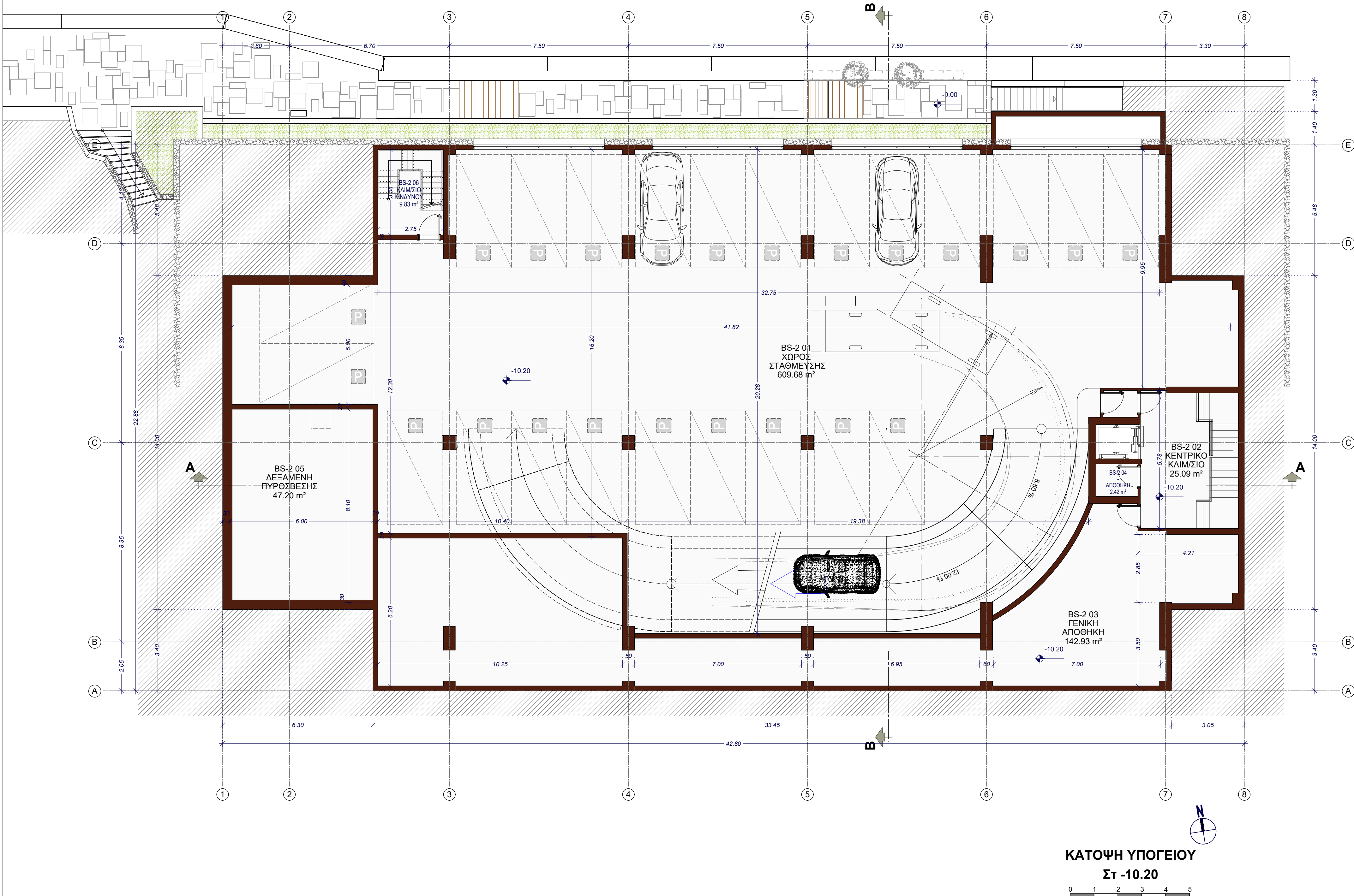
ΠΡΟΟΠΤΙΚΗ ΑΠΟΨΗ 2ου ΥΠΟΓΕΙΟΥ (Χώρος Στάθμευσης)
