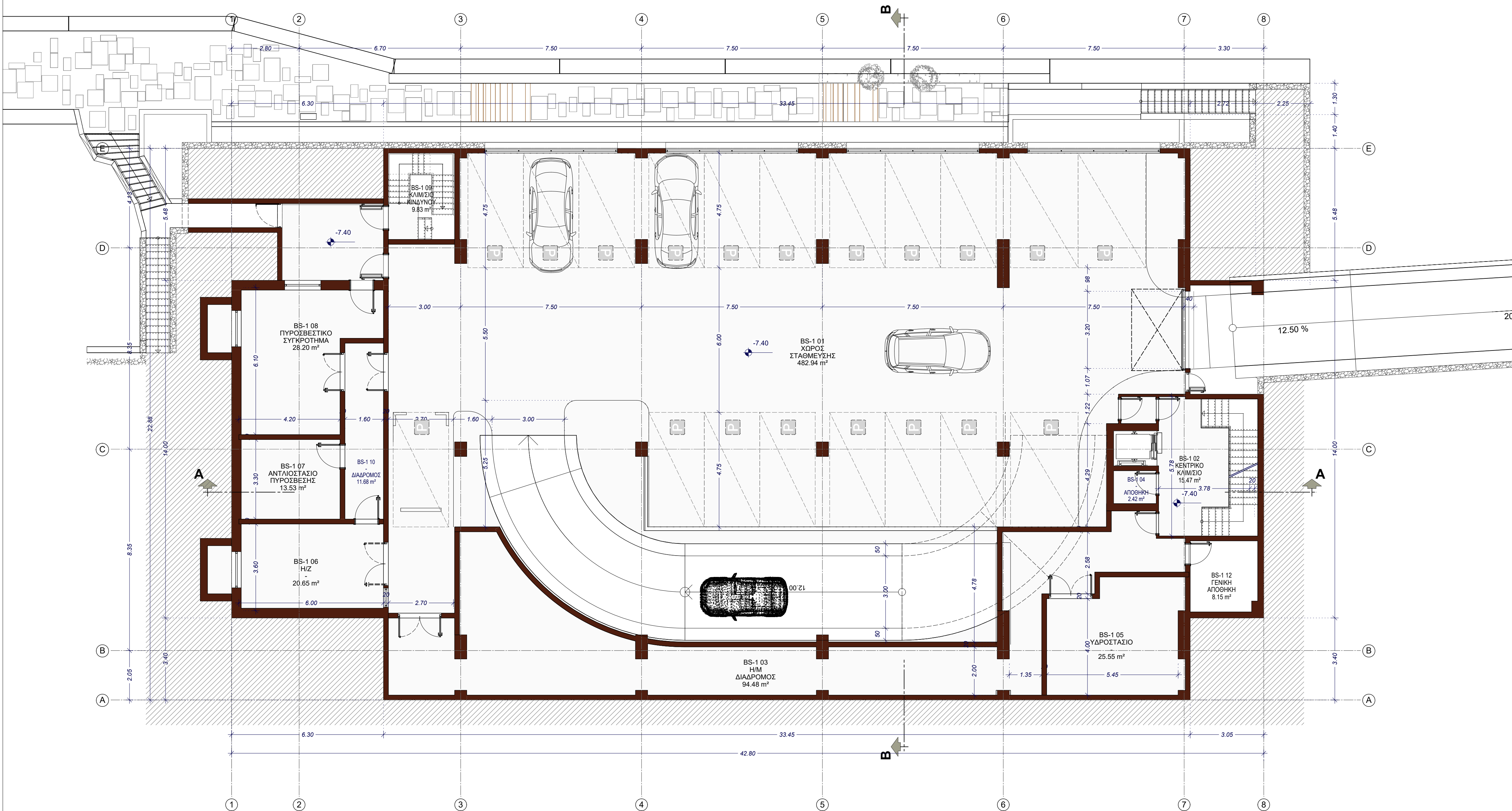
ΚΑΤΟΨΗ ΥΠΟΓΕΙΟΥ ΣΤ -7.40
