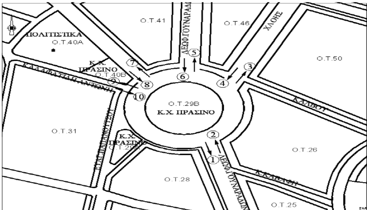
Σχήμα 1 Αρίθμηση στρεφουσών κινήσεων οχημάτων στον κόμβο Κ19
