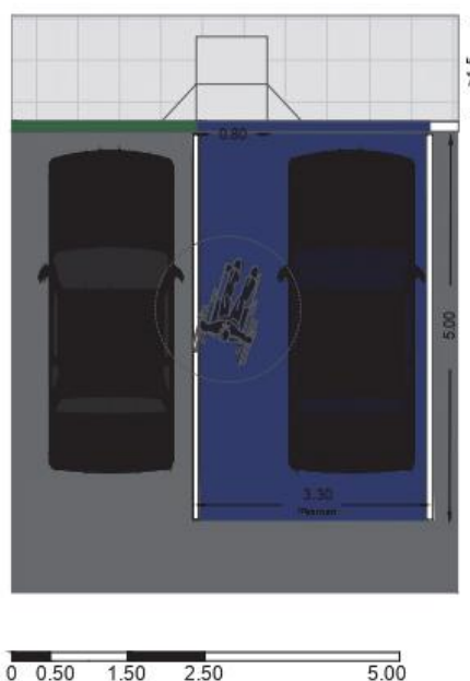
Σκαρίφημα προτεινόμενης θέσης στάθμευσης ΑμεΑ (κατά ΣΧ.26.Α - ΘΕΣΗ ΣΤΑΘΜΕΥΣΗΣ ΑμεΑ ΚΑΘΕΤΑ ΣΤΟ ΠΕΖΟΔΡΟΜΙΟ, Παράρτημα της ΥΑ ΥΠΕΝ/ΔΜΕΑΑΠ/124964/1561/2022)
